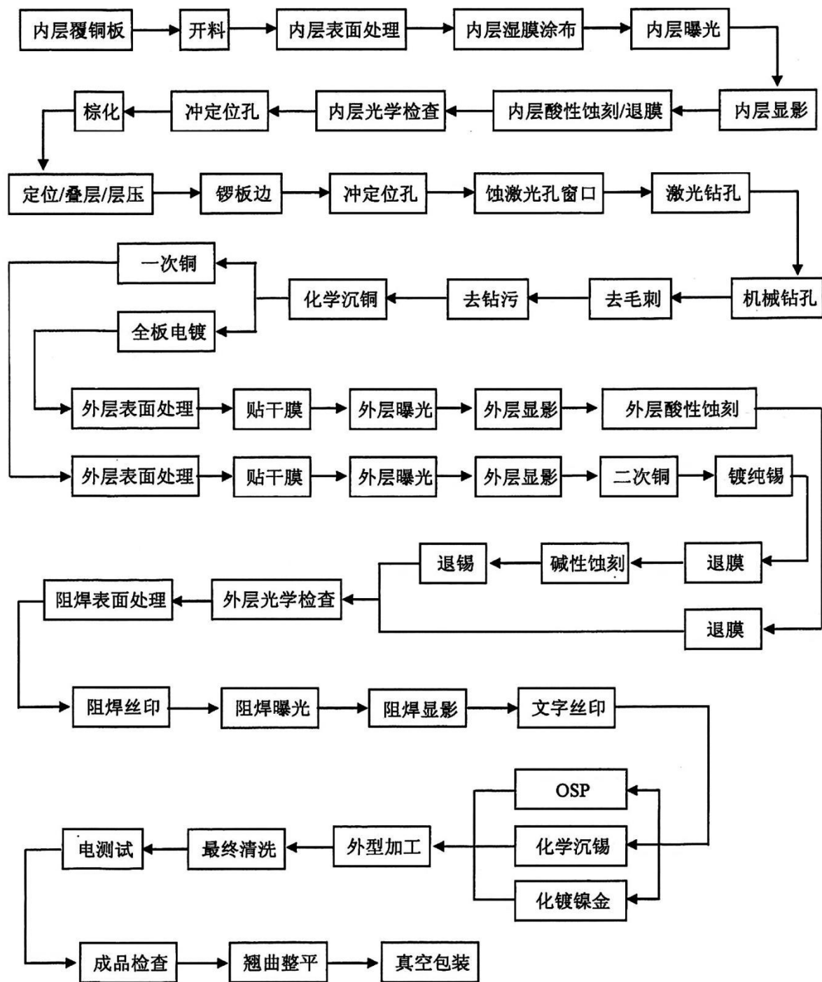
图1 印制线路板生产工艺流程及产污环节图
