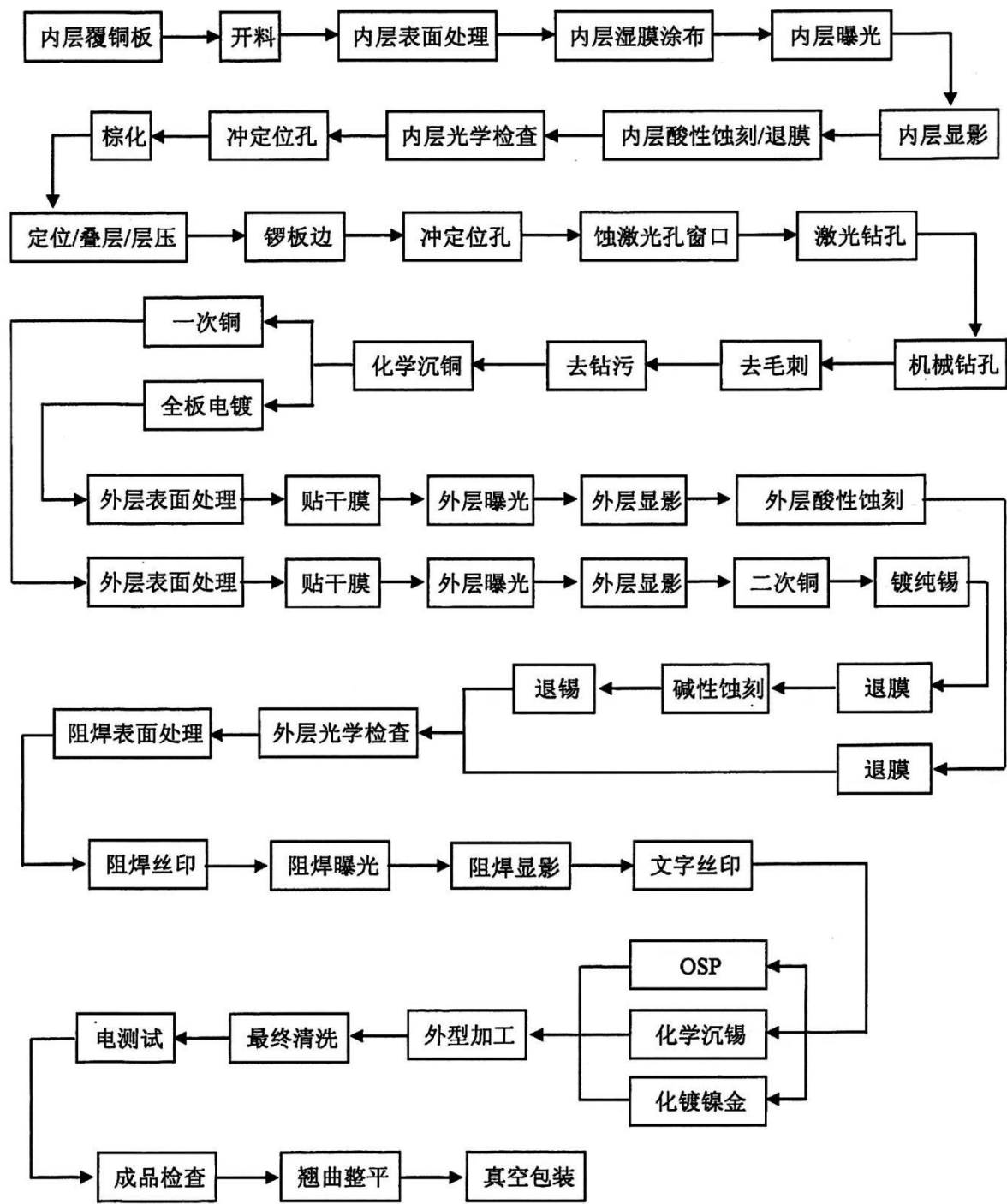
图 1 线路板生产工艺流程及产污节点图
